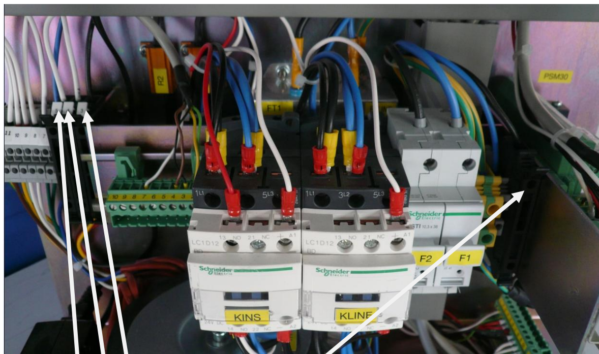
Fusible F5 – F4- F3 (6,3AT) et Fusible de 2,5 AT sur alimentation 12Vdc du split box.
