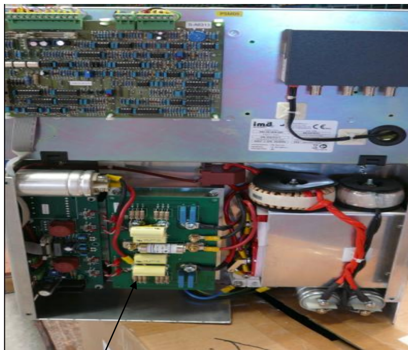
PSM 03 et son fusible de 80 A 660V
