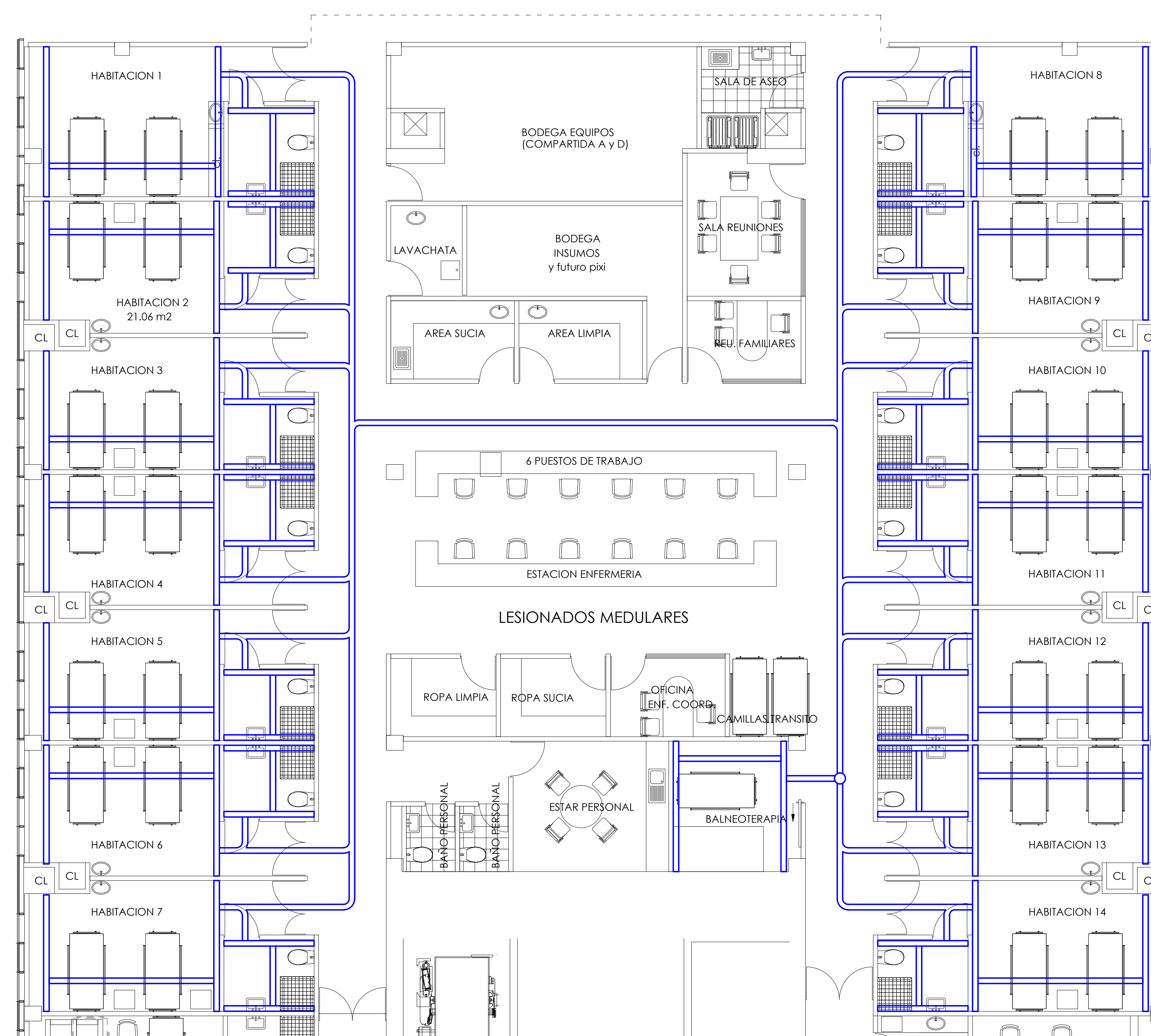
PLANTA HABILITACION PISO 4 EDIFICIO D_AREA REHABILITACION PROYECTO LEVANTADOR DE PACIENTES, GULDMANN ESC. 1_100
