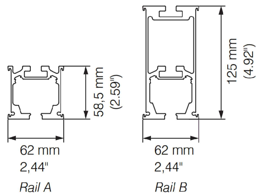
DETALLE RIELES ESC. S/ESC
