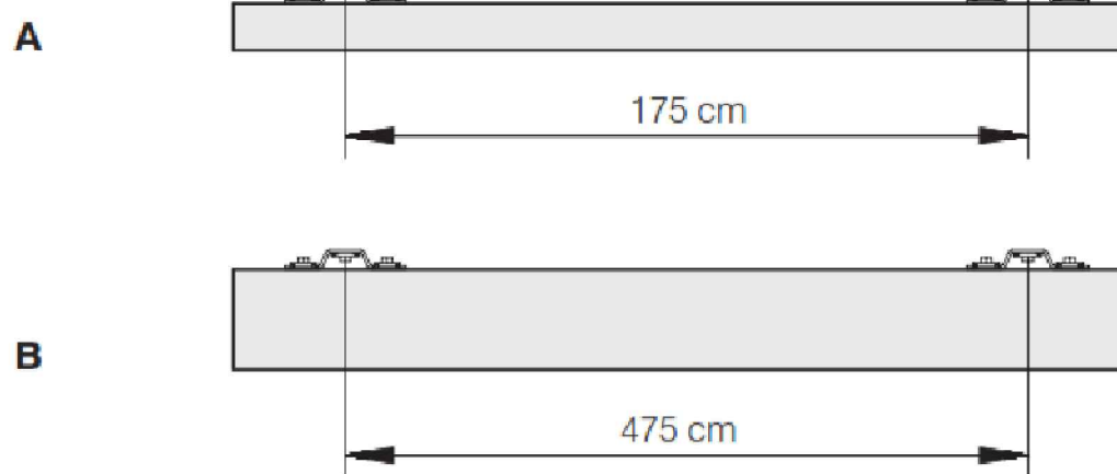
DETALLE DISTANCIAS MAXIMAS ENTRE ANCLAJES ESC. S/ESC
