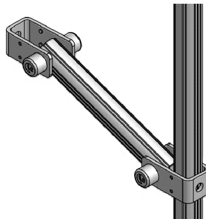
DETALLE ESTABILIZADOR DE ANCLAJE A LOSA ESC. S/ESC
