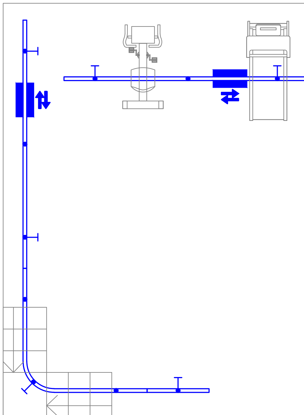
PLANTA RIELES TRASLADO DE PACIENTE SIN ESC.
