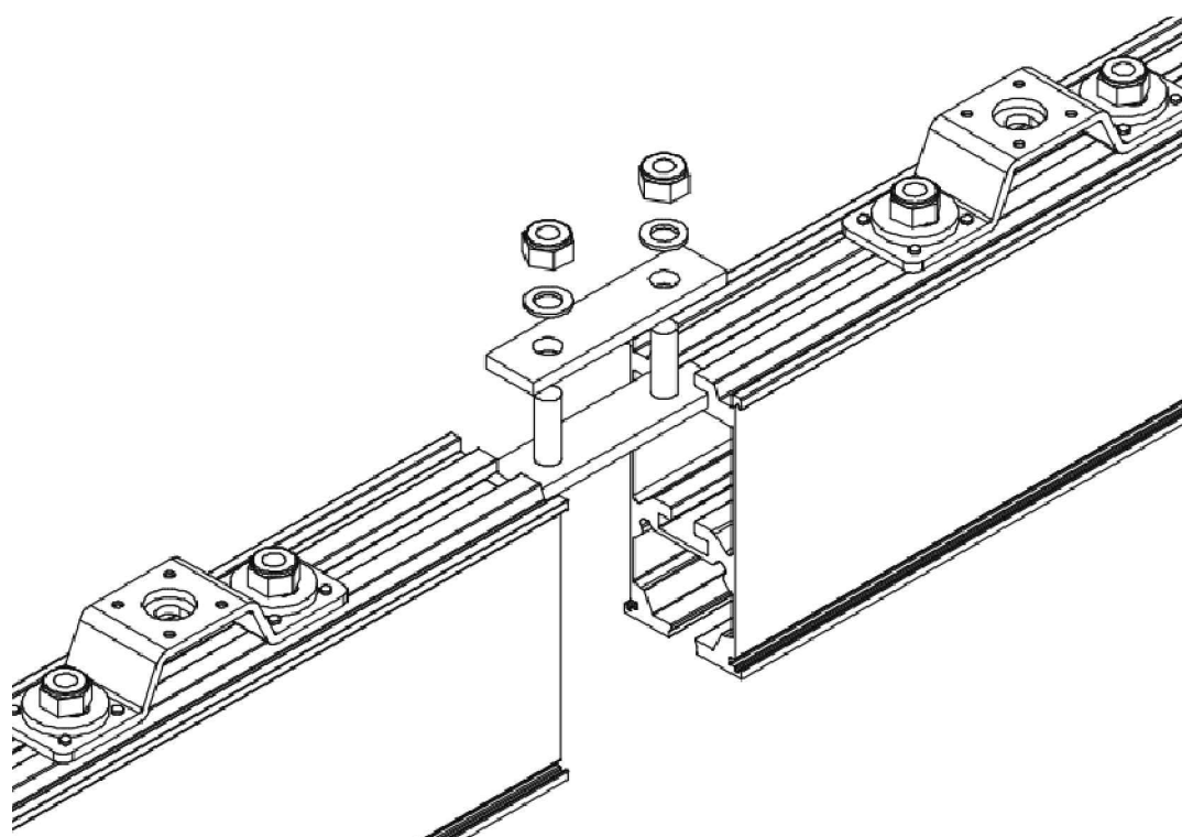
DETALLE ACOPLES DE RIELES TIPO ESC. S/ESC
